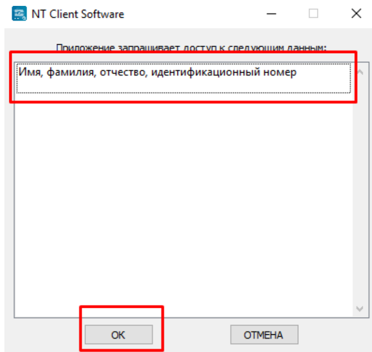
Рисунок 3. Окно КП
